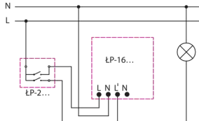
Układ realizuje funkcję: Zawsze włączony (czujnik ruchu odłączy od układu) Sterowanie czujnikiem, Zawsze wyłączony
